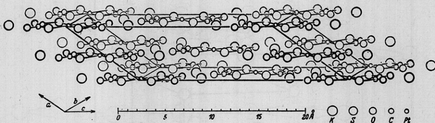
FIG. 7. The structure of K_2[Pt(C_2O_2S_2)_2] ( Strukturbericht )
